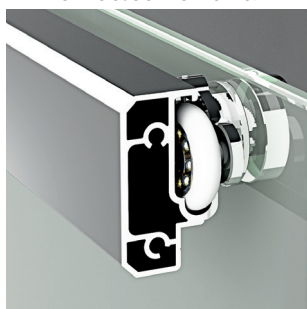
Doble Rodamiento regulable con dispositivo antidescarrilamiento.
