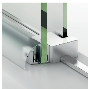
Guía Inferior con dispositivo de liberación de Puertas
