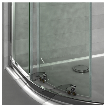
Detalle rodamientos
