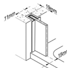
Detalle perfil empotrado de 8mm
