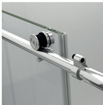
Detalle rodamiento y limitador de recorrido
