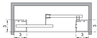
Detalle cierre 2P
