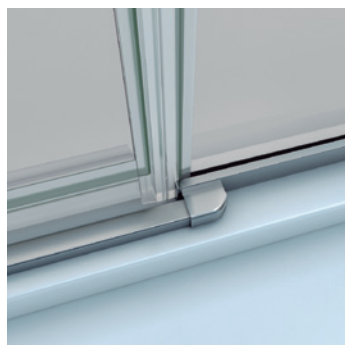
Detalle junquillo de estanqueidad
