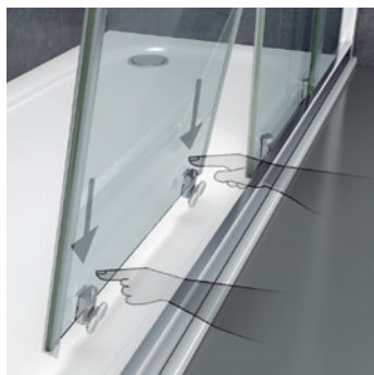
Detalle liberación de puertas.
