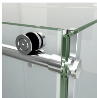
Detalle unión de cerco a lateral
